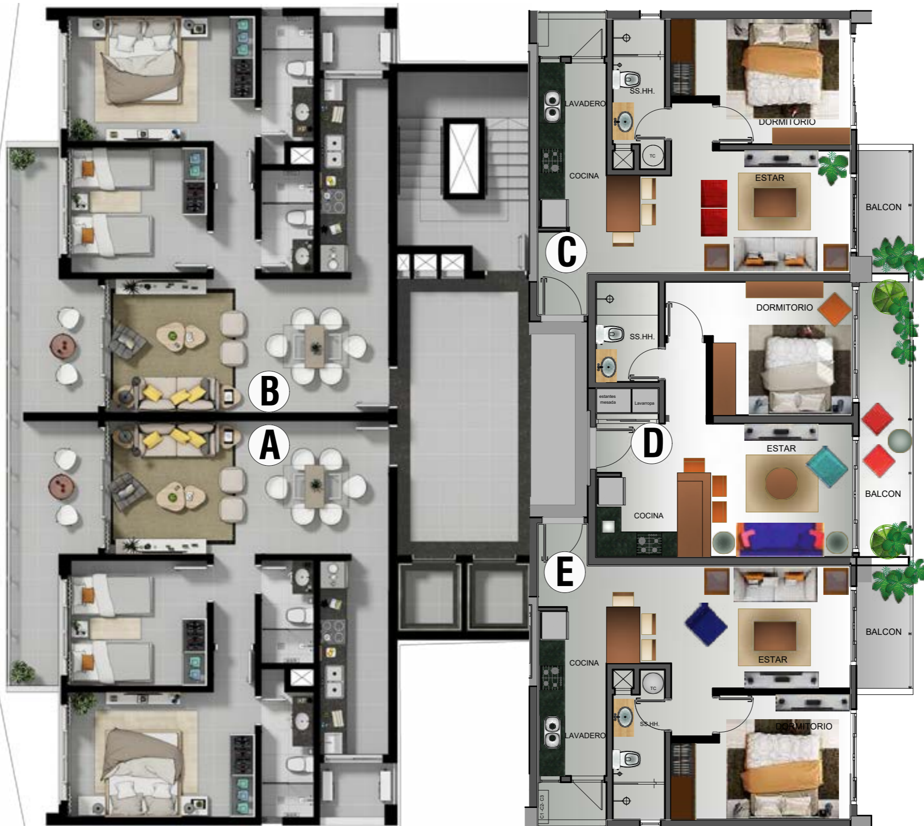
PLANTA TIPO DEPARTAMENTOS DE 1 Y 2 DORMITORIOS -CON EQUIPAMIENTO REFERENCIAL SIN ESCALA
